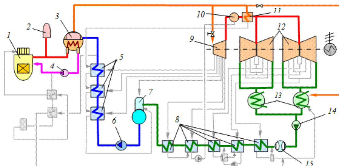
Рис. 1. Принципиальная тепловая схема энергоблока АЭС с реактором ВВЭР-1000: 1- реактор; 2- компенсатор объема; 3- парогенератор; 4- ГЦН; 5- подогреватель высокого давления; 6- питательный насос; 7- деаэратор; 8 – подогреватели низкого давления; 9 – ступени высокого давления турбины; 10 – сепаратор; 11- пароперегреватель; 12 – ступени низкого давления турбины; 13 – конденсаторы; 14- конденсатный насос; 15 - эжекторы.
