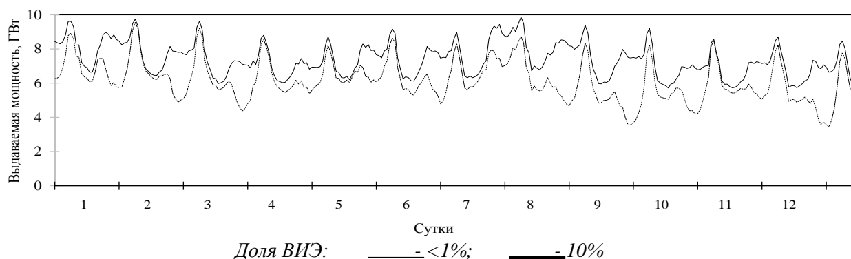
Рис. 4. Загрузка тепловых электростанций при разной доле ВИЭ в выработке электроэнергии в энергосистеме
