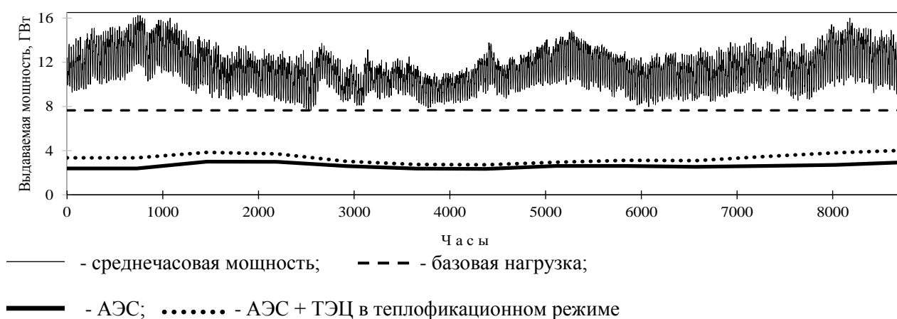
Рис. 1. Среднечасовая мощность электростанций энергосистемы Юга в 2017 г.
