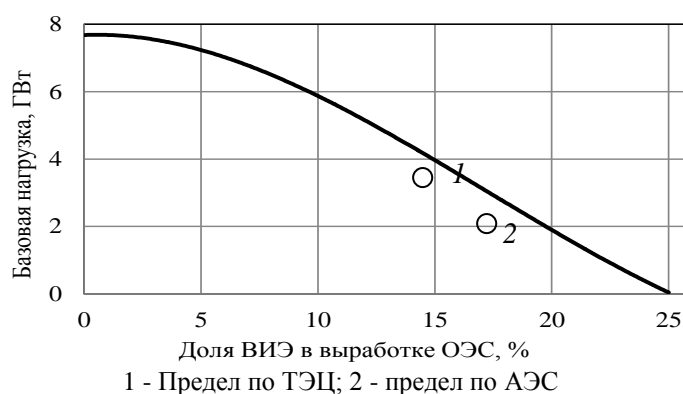
Рис. 3. Зависимость базовой нагрузки энергосистемы Юга от доли электростанций на ВИЭ.
