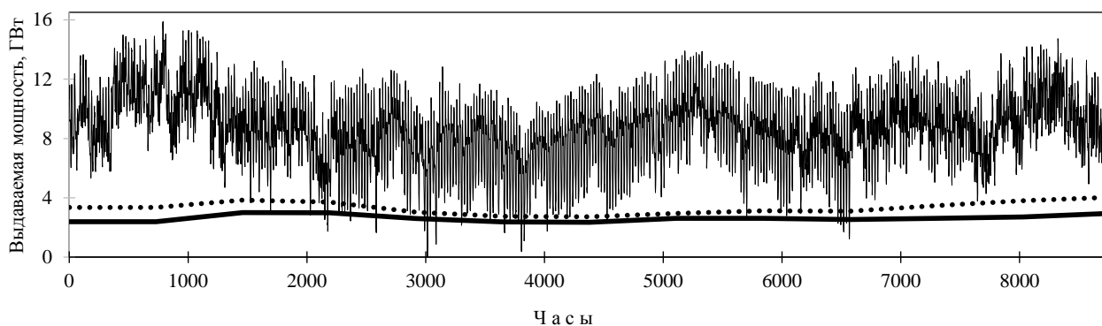
Рис. 2. Потребность в мощности традиционных электростанций в энергосистеме Юга при доле ВИЭ в выработке электроэнергии равной 25% (Обозначения - см. рис. 1)
